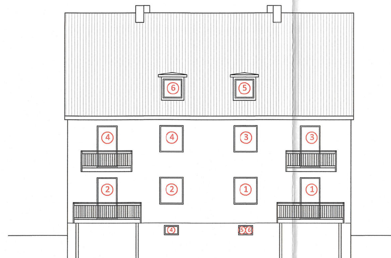
RÜCKANSICHT
