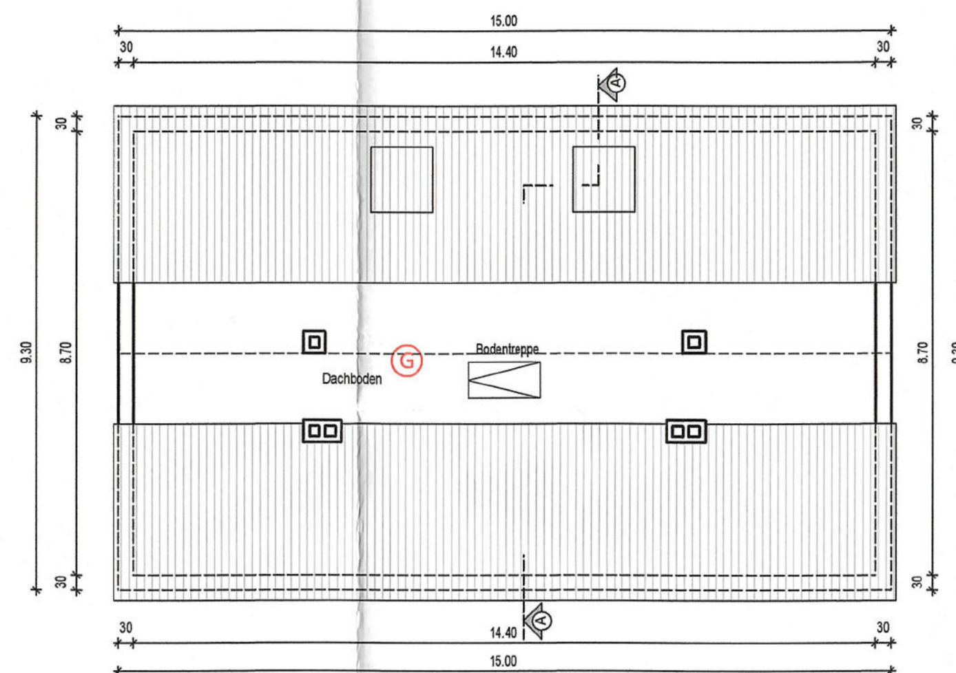
DACHBODEN
