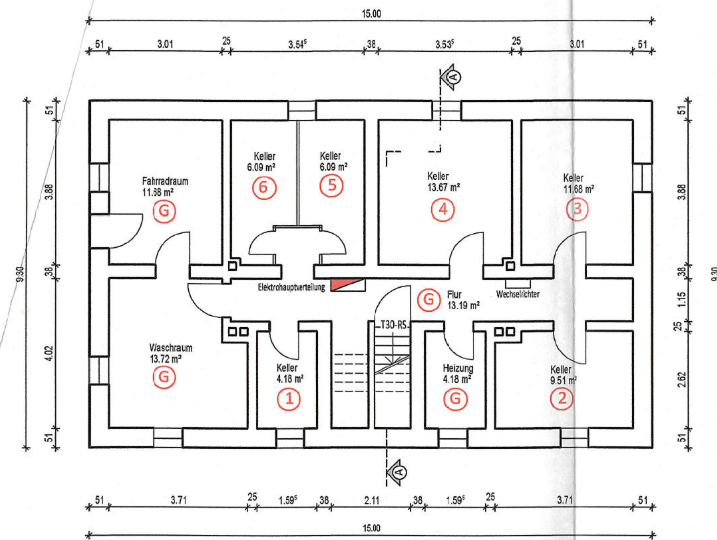
KELLERGESCHOSS
