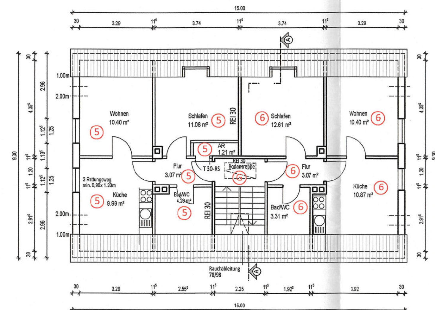
DACHGESCHOSS
