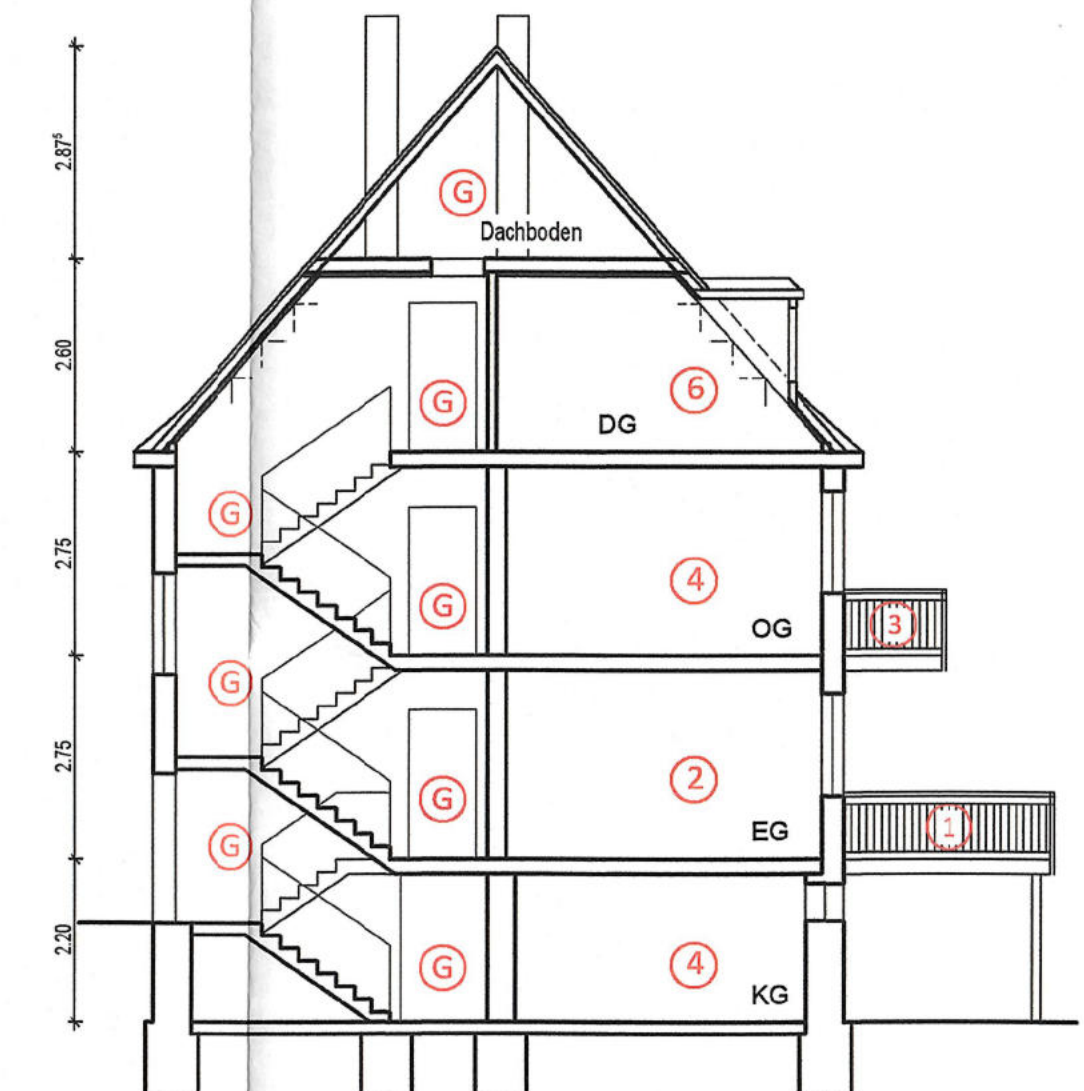
SCHNITT A-A
