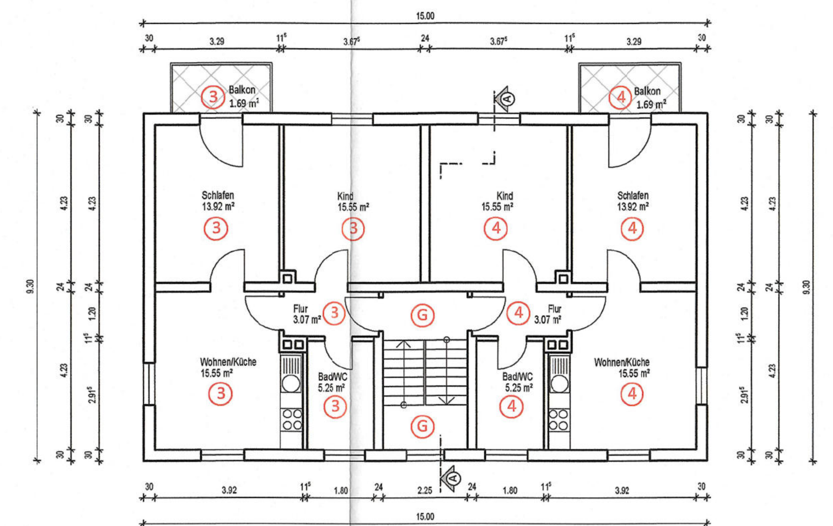
OBERGESCHOSS
