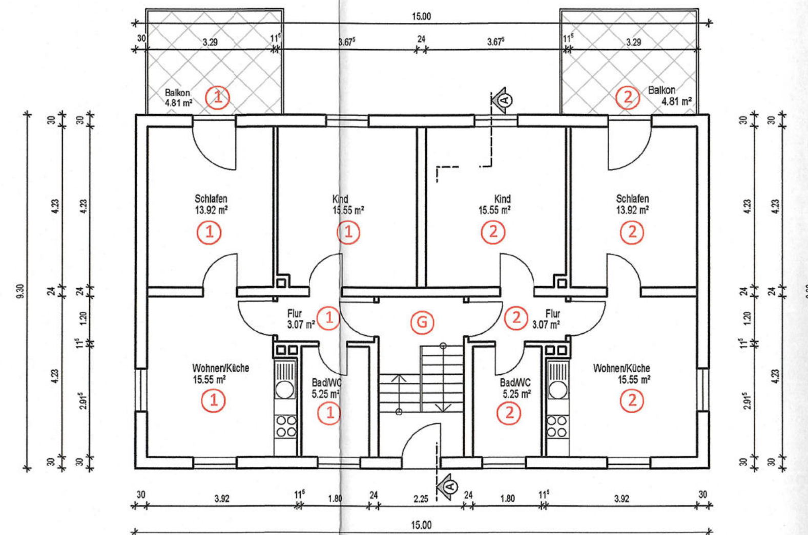
ERDGESCHOSS
