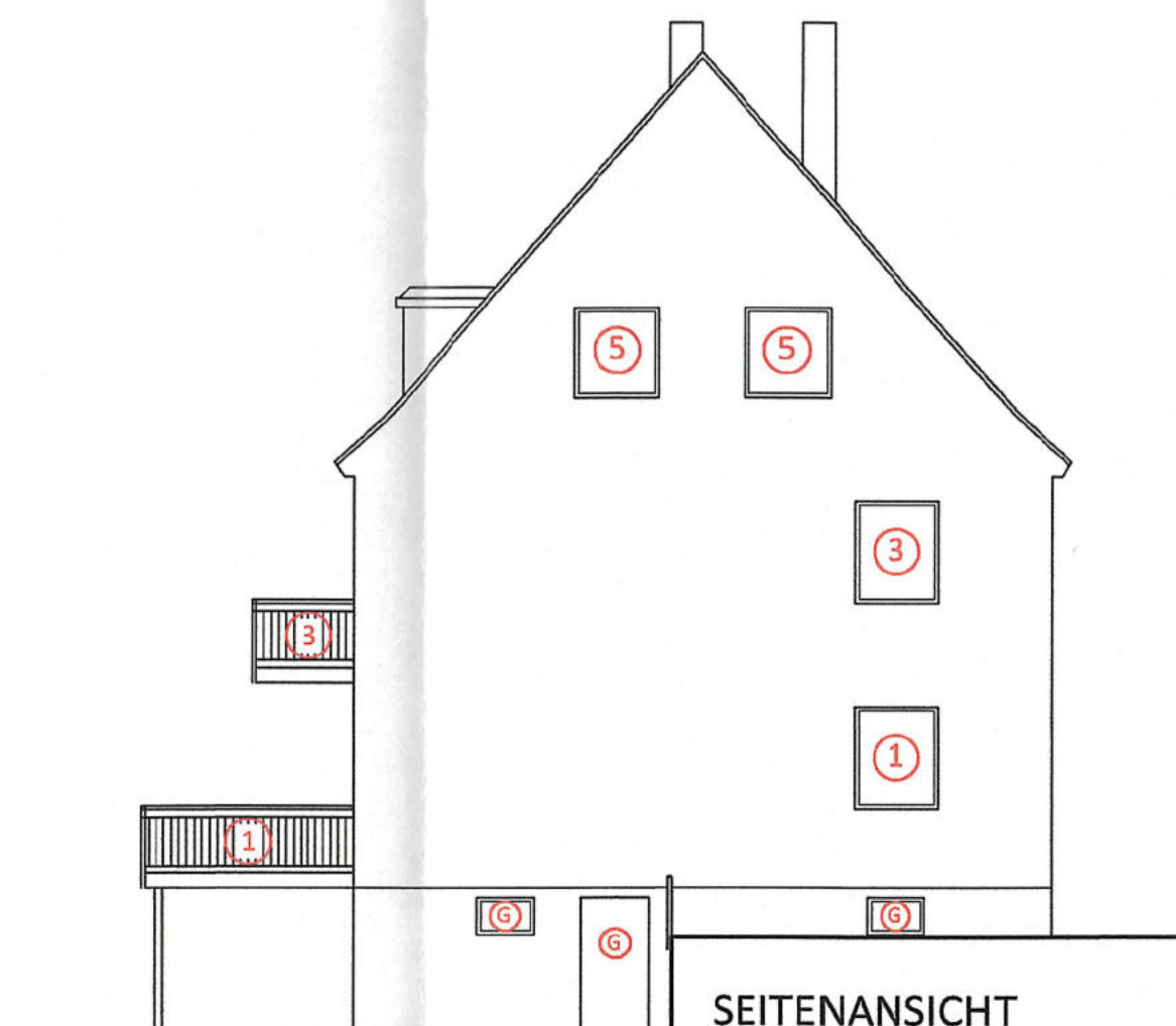
SEITENANSICHT
