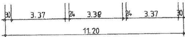
OBERGESCHOSS (BESTAND)
