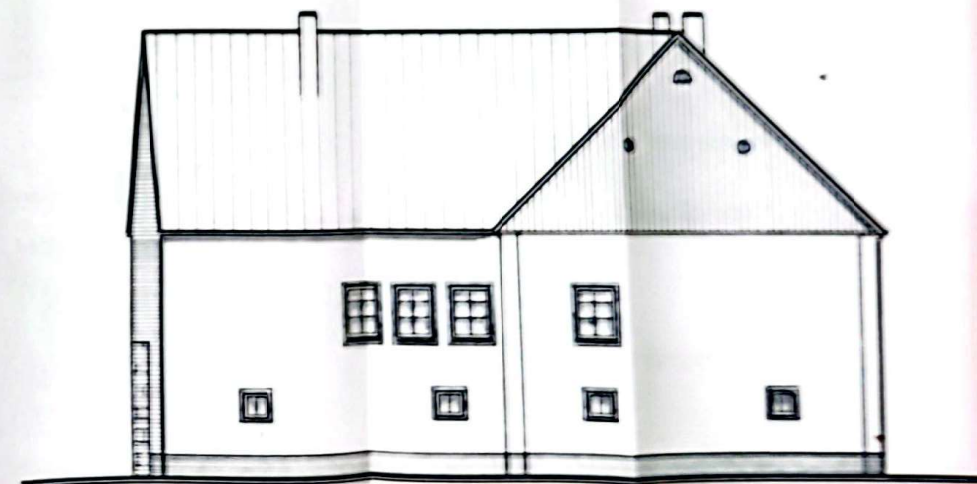
SEITENANSICHT-RECHTS
