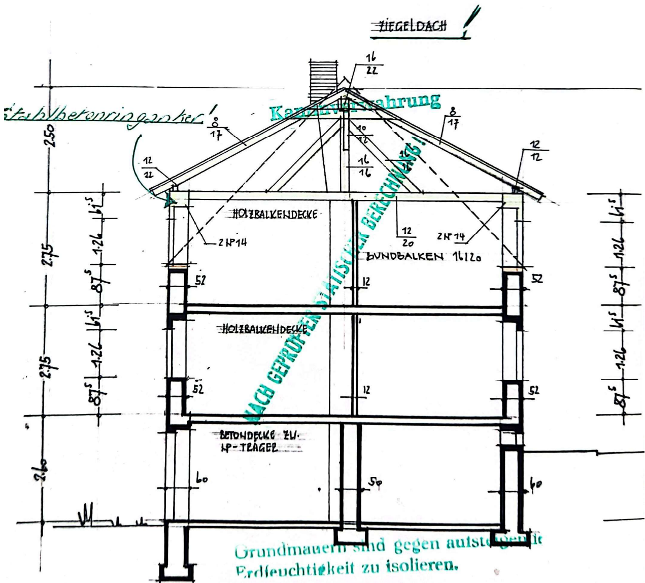
QUERSCHNITT (AUFSTOCKUNG)
