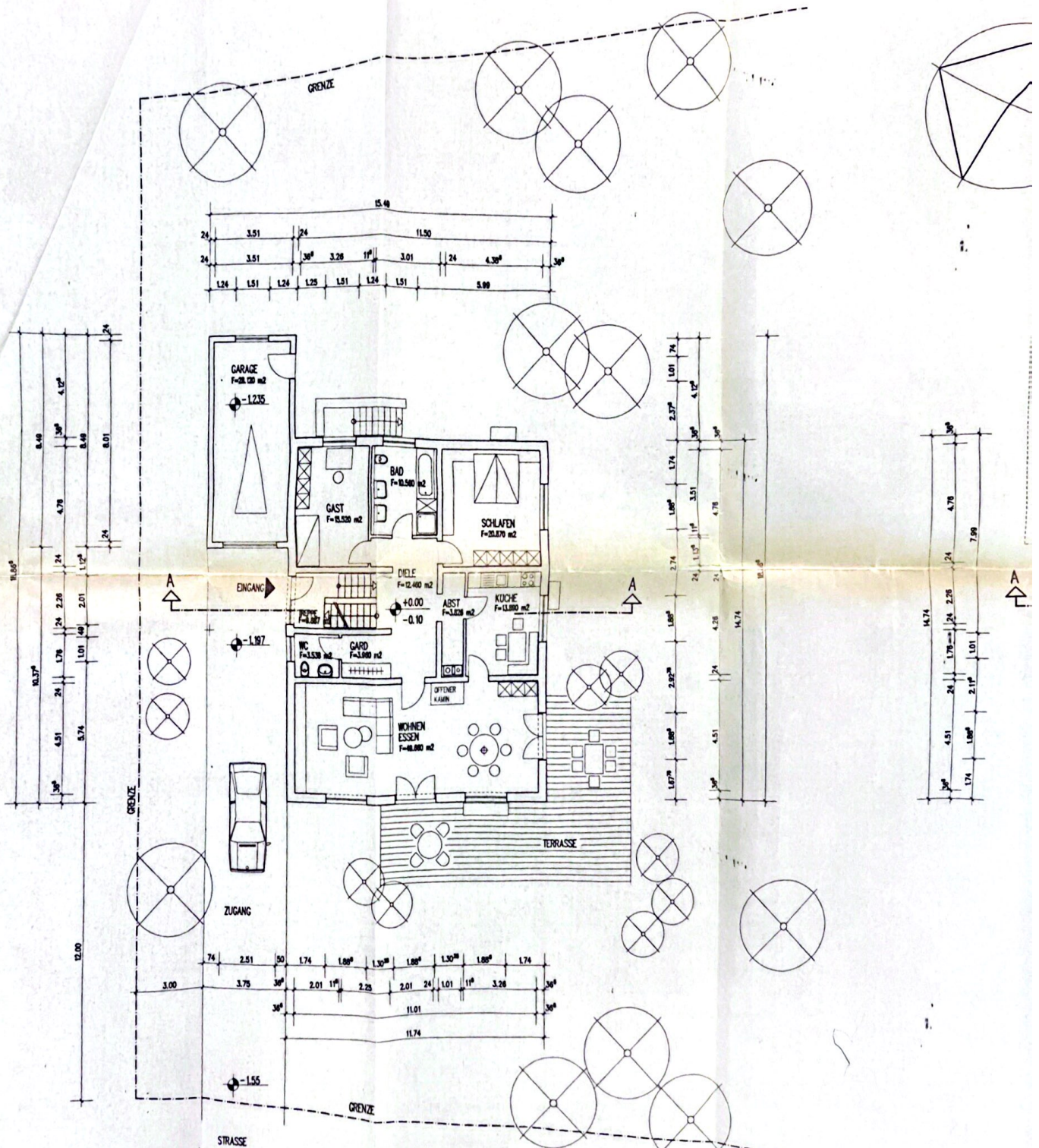
GRUNDRISS ERDGESCHOSS
